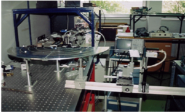
Διάταξη μέτρησης ΟΠΤΙΚΩΝ ΙΝΩΝ
